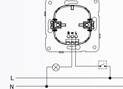
Merkezi Anahtar ile Kullanım
