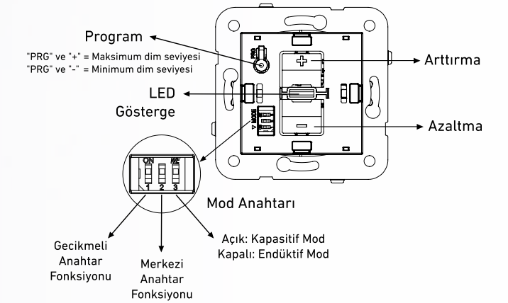
Merkezi Anahtar ile Kullanım
